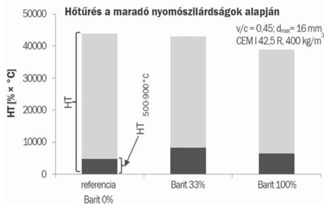
13. ábra A 0/6 mm-es barit adagolás hatása a beton nyomószilárdságának hőtürése (jelölés: barit adagolás m/m 0/4 -ban)
