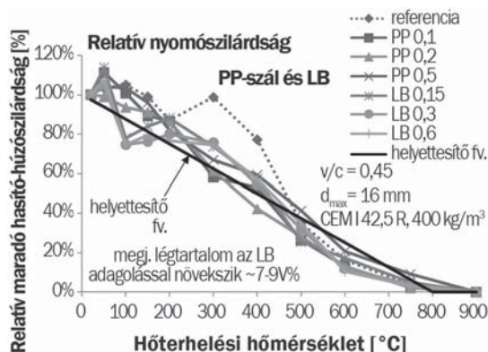
7. ábra A PP-szál és légbuborék-képző adalékszer adagolásának hatása a beton hőterhelés utáni relatív maradó nyomószilárdságára (jelölés: PP-szál adagolás V/V%; LB adagolás m/m 3 )
