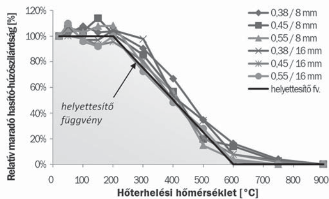
4. ábra A víz/cement tényező és a maximális szemnagyság hatása a hőterhelés utáni relatív maradó hasító-húzószilárdságra (jelölés: víz/cement tényező / maximális szemnagyság) Fig. 4. Effect of the water/cement ratio and maximal grain size on the relative residual split-tensile strength (notation: water/cement ratio / maximal grain size)
